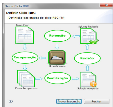
Figura 1 – Execução do Ciclo do RBC
